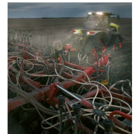
▲ Lielākā hidrauliskā sistēma ar līdz pat 537 l/min un astoņiem hidroizvadiem nodrošina augstāko elastības un efektivitātes līmeni tirgū.
