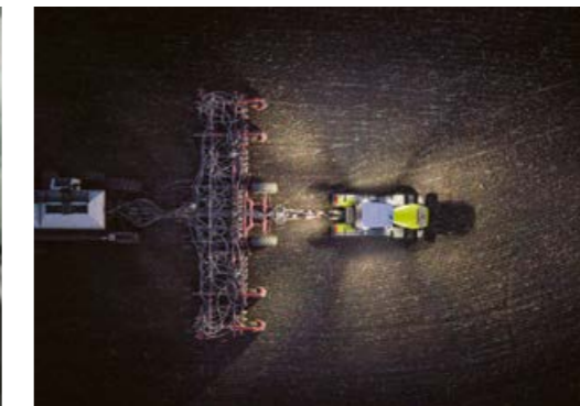
◀ Augstākās klases apgaismojuma komplekts ar līdz pat 22 LED priekšējiem lukturiem nodrošina 53 400 lm, lai darba zona tiktu apgaismota 360° rādiusā.
